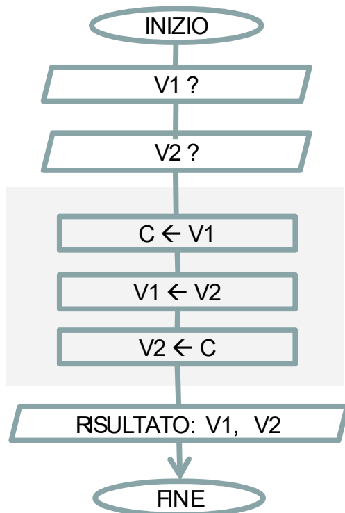
Algoritmo
